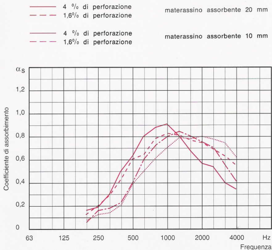
fig. 2 Materassini fonoassorbenti Idikell M protetti con membrana perforata tesa. Coefficiente di assorbimento in funzione della frequenza.
