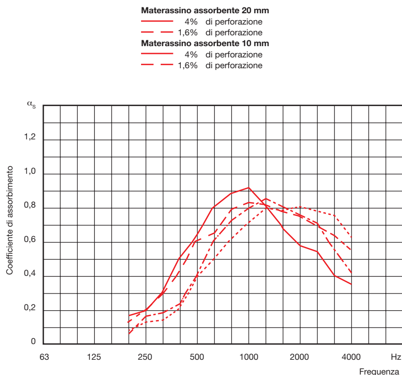
Fig. 2 - I Materassini fonoassorbenti Alfakel M6000 protetti con membrana perforata tesa. Coefficiente di assorbimento in funzione della frequenza.
