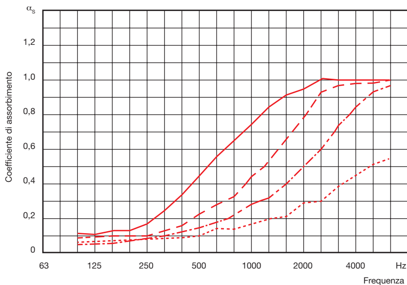
Fig. 1 - Materassini fonoassorbenti Alfakel M6000. Coefficiente di assorbimento in funzione della frequenza.
